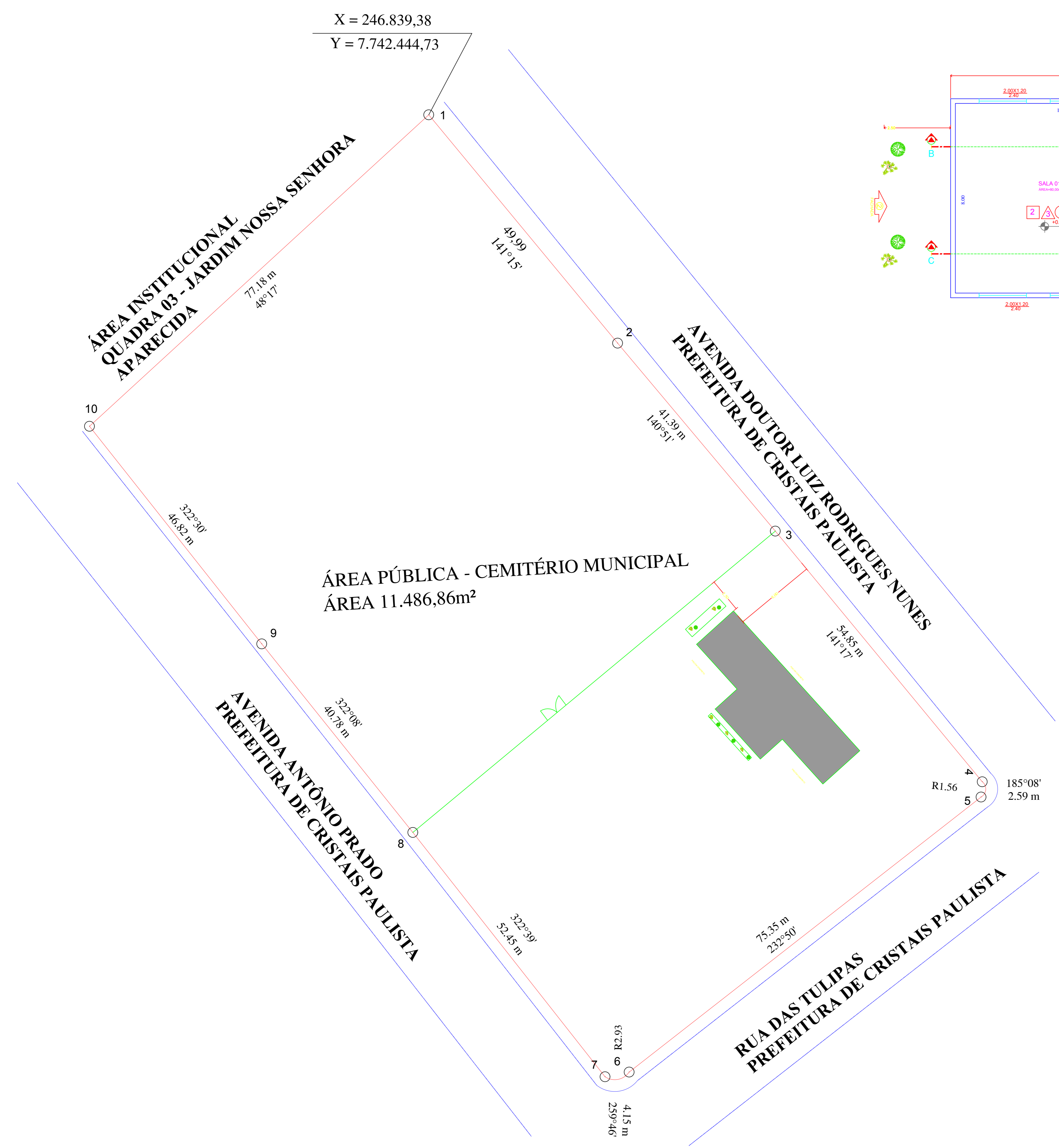
PLANTA DE IMPLANTAÇÃO Escala 1:200
